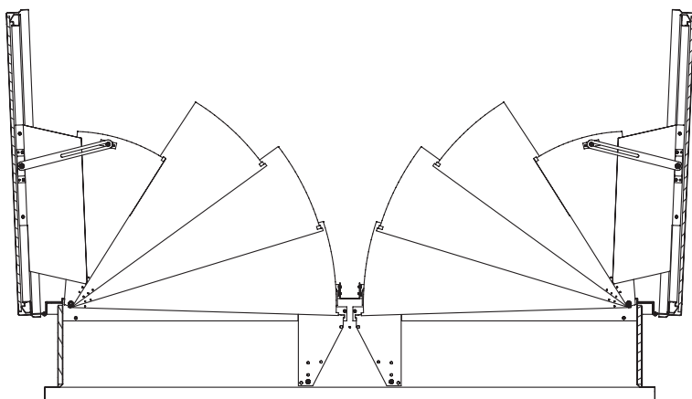
Hexacoif DoE Eventail nyitott pozícióban
