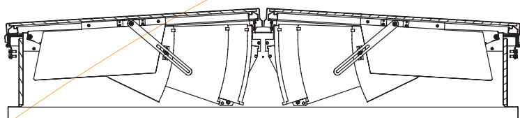
Hexacoif DoE Eventail zárt pozícióban
