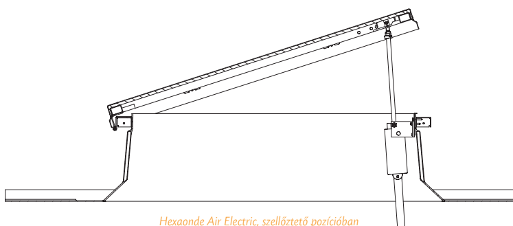
Hexaonde Air Electric, szellőztető pozícióban
