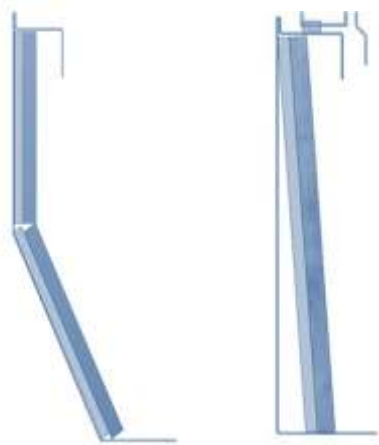
Acél lábazat 25 mm hőszigetelés
