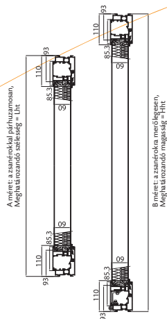
Hangszigetelt héjalás
