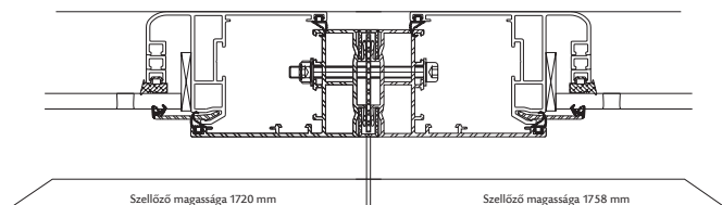
Két keret összeillesztése
