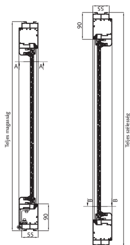
Üveg héjazat
