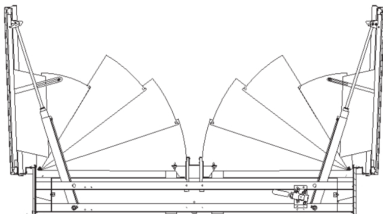
Hexasteel DoP Eco nyitott pozícióban – 90° nyitási szög
