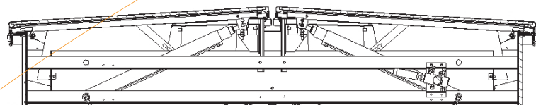
Hexasteel DoP Eco zárt pozícióban
