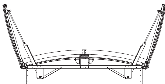
Hexavoûte DoP nyitott pozícióban
